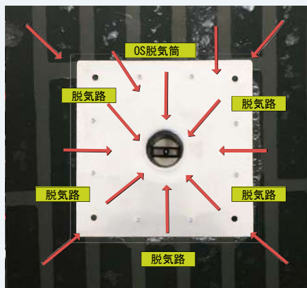
裏から見たOS-sheets脱気システム(OS-Z40)
