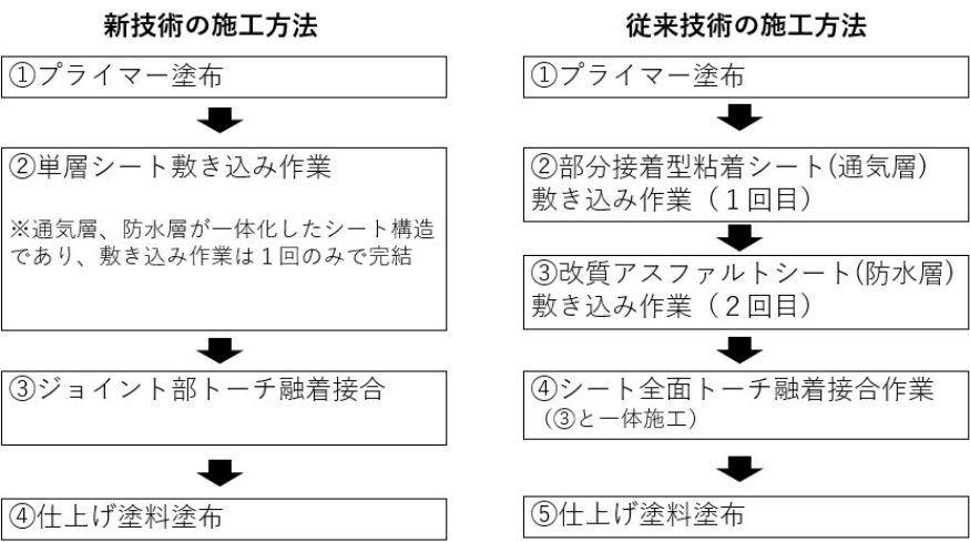
各技術の施工手順比較図
