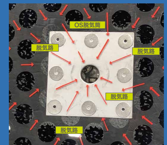
裏から見たOS-sheets脱気システム (OS-Z40)
