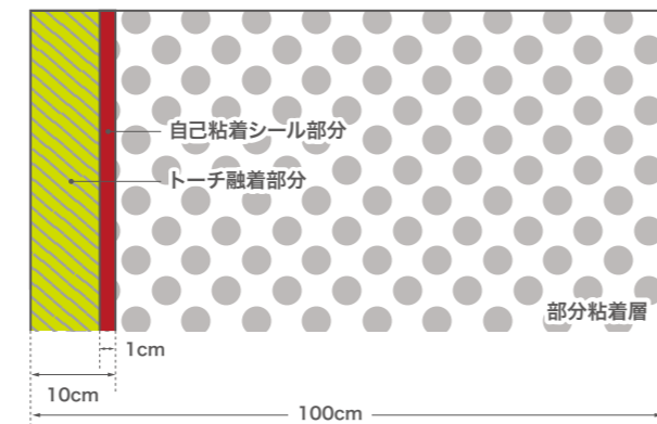
OS-sheets 裏面 (上側シート)
